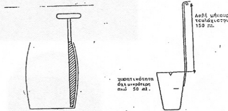
Σχήμα 3: Αναθεωρημένος κατάλληλος για την ανάλυση της αεροσυσσωματωμένου γάλακτος
