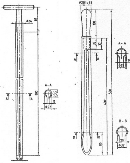
Σχήμα 5: Δειγματολήπτες για γάλα σε σκόνη (όλες οι διαστάσεις σημειώνονται σε mm).
